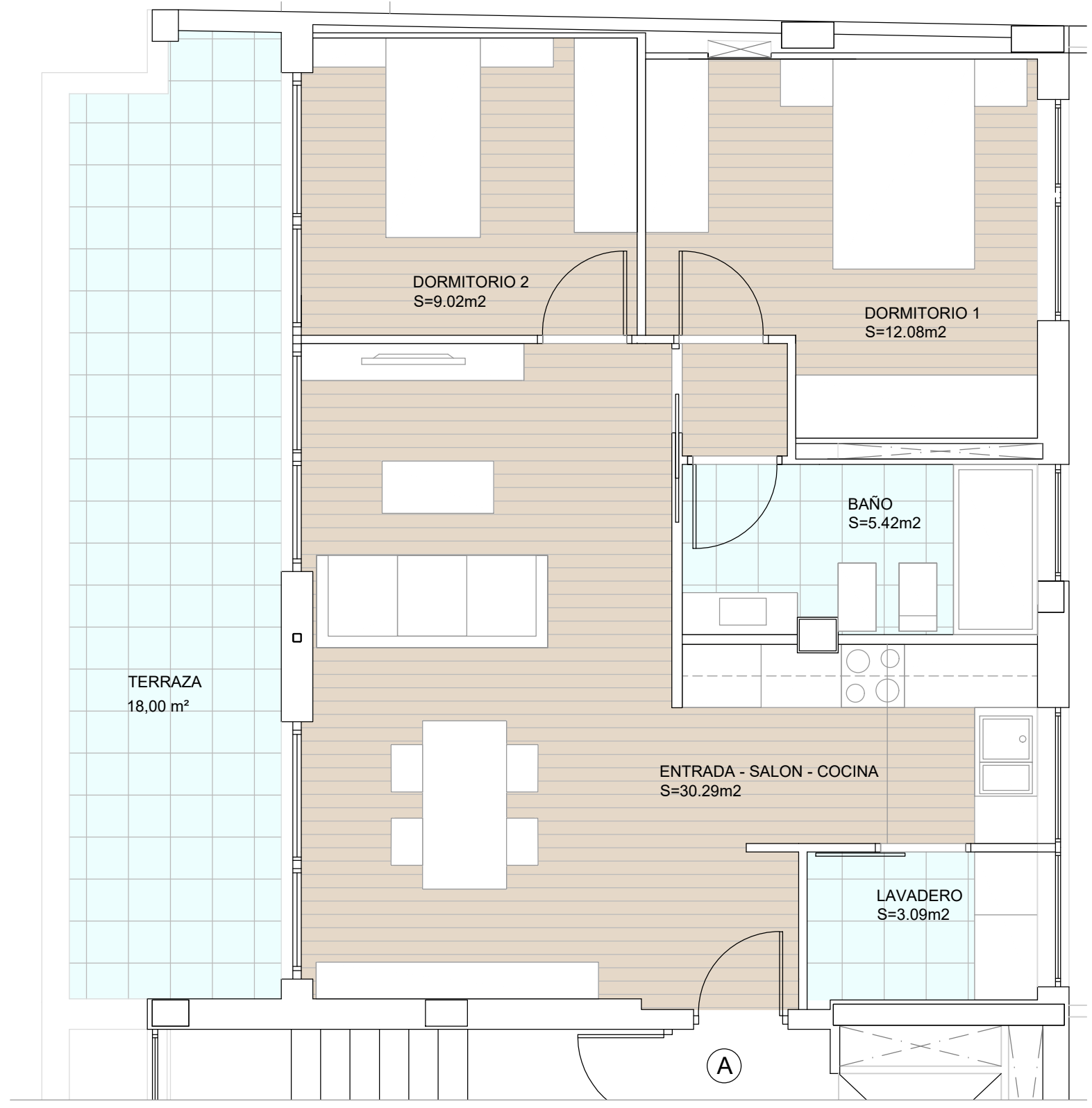
PLANTA BAJOCUBIERTA-A (2 DORMITORIOS) ESCALA 1/50
